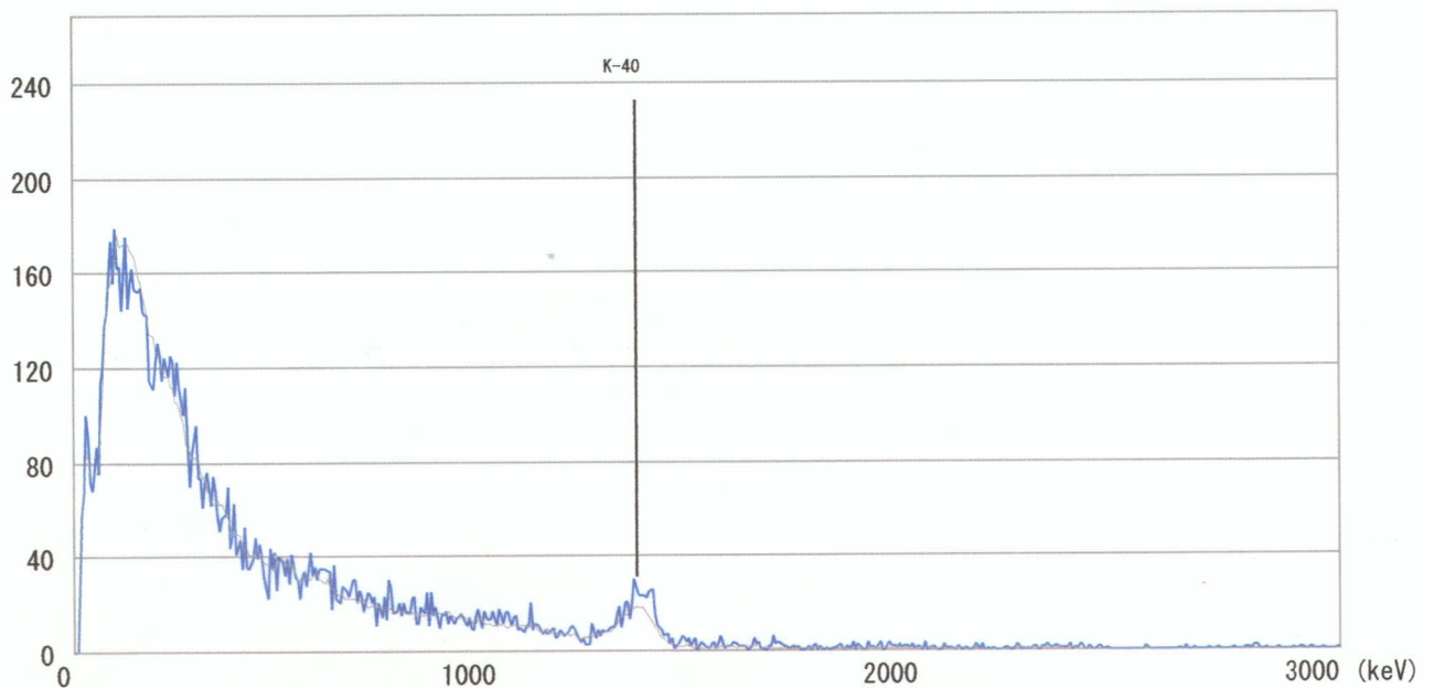
スペクトル解析結果 (データID: 1216)
