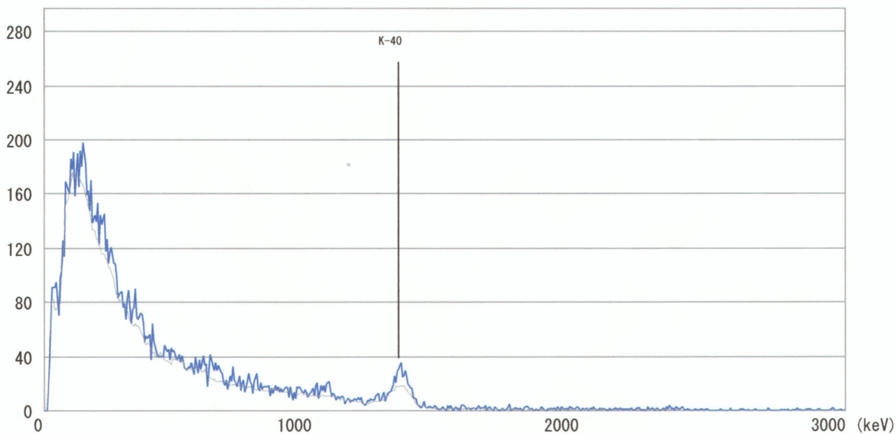
スペクトル解析結果 (データID: 2035)
